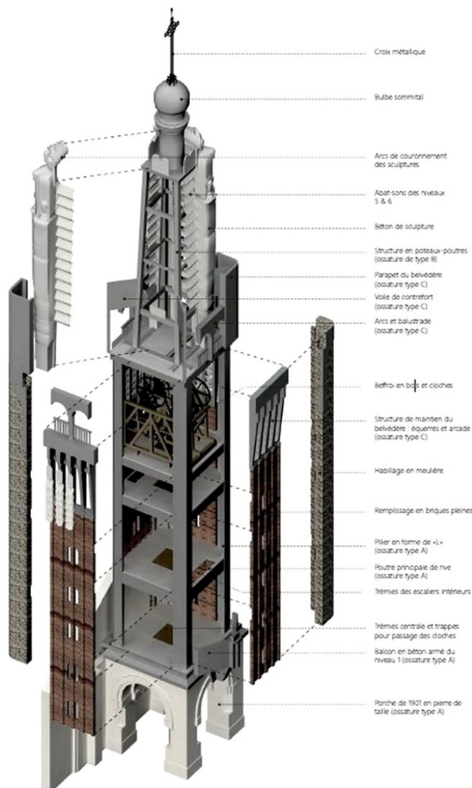
Modélisation 3D de la structure - Atelier Ergon
